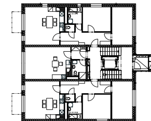
PŮDORYS 1. NP umístění bytu v rámci podlaží
