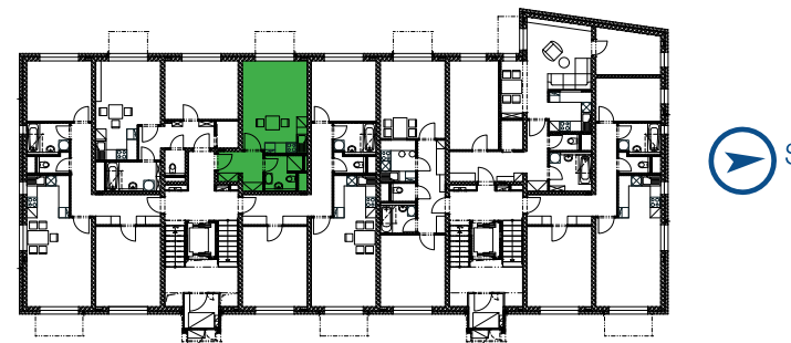
PŮDORYS 1. NP umístění bytu v rámci podlaží
